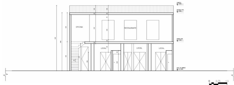
Corte longitudinal
